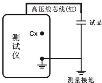
图 12 反接法
