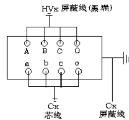
图 12 变压器接法
