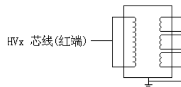
图7 PT接法
