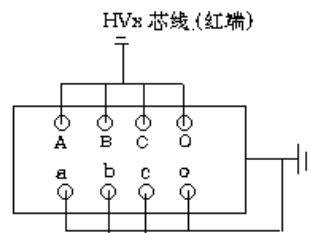
图 13 变压器接法
