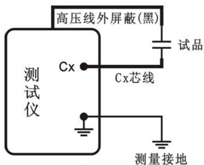
图 11 正接法
