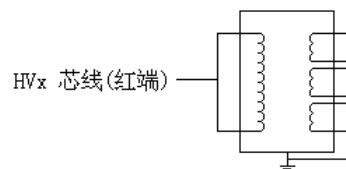
图10 CT接法
