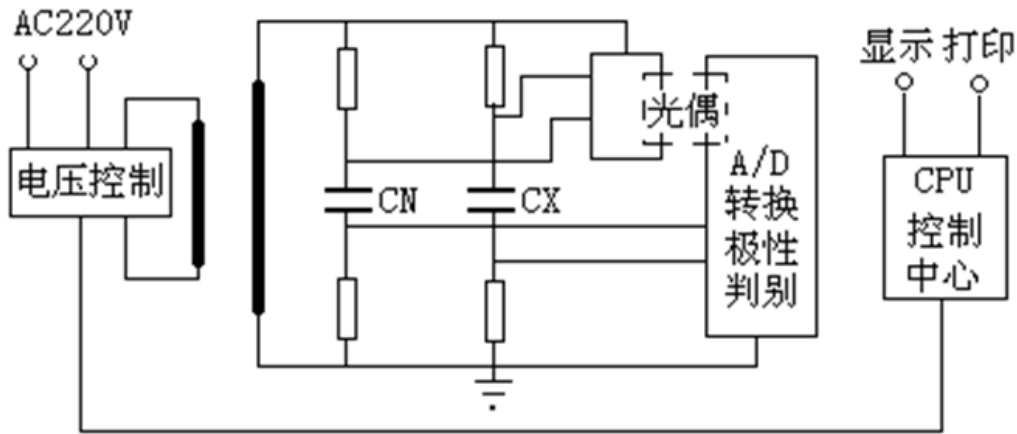
图 1 测量原理图
