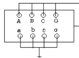
图 14 变压器接法
