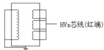
图8 PT接法
