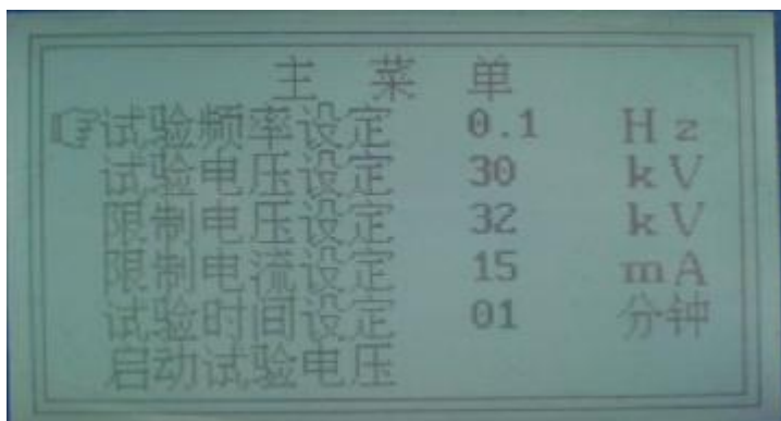
图4 (设定界面)
