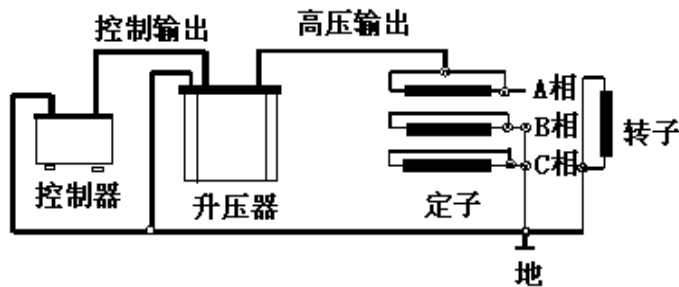
图 8 测量定子的某相连线图
